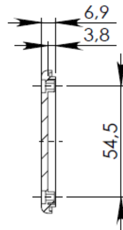
PRZEKRÓJ A-A
