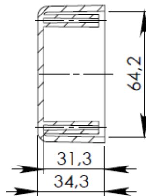
PRZEKRÓJ B-B
